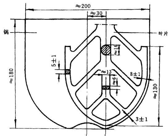
图 1 搅拌机
