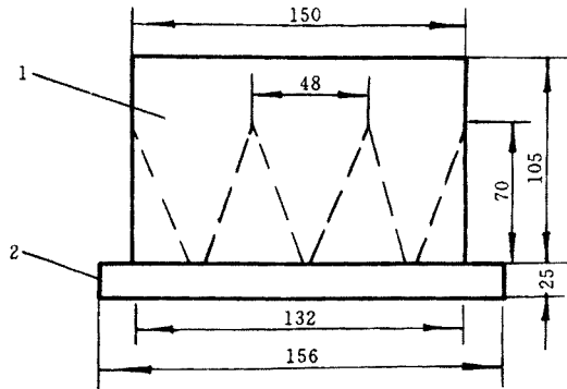
1—漏斗;2—模套
