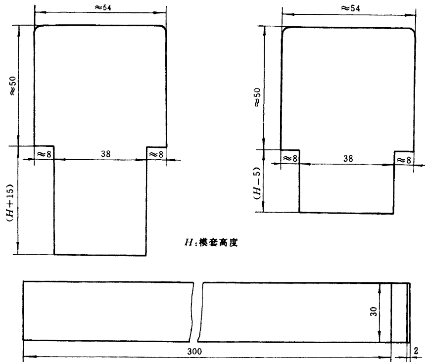
图 3 典型的播料器和金属刮平尺
