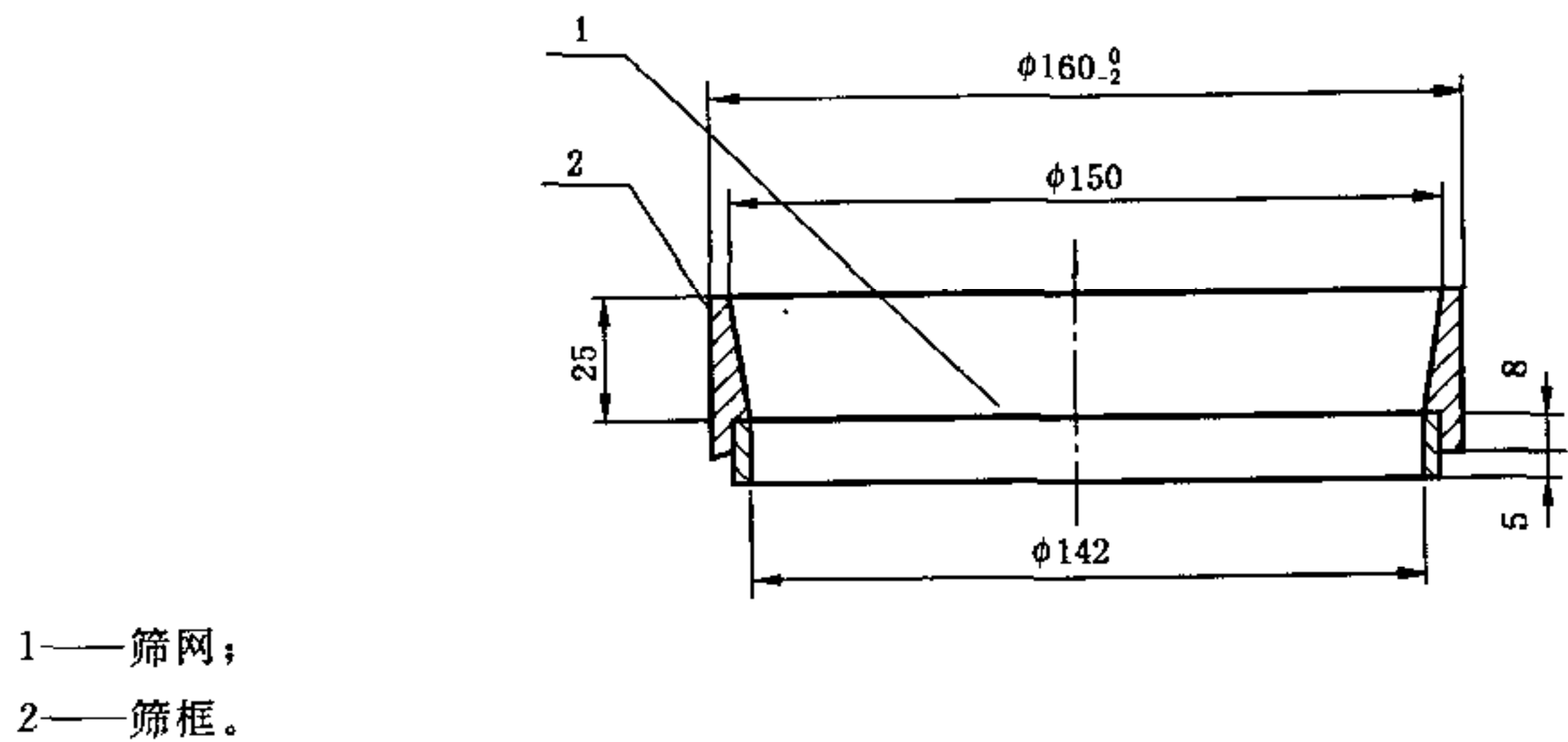
图 A.1 45 \mu\text{m} 方孔筛示意图
