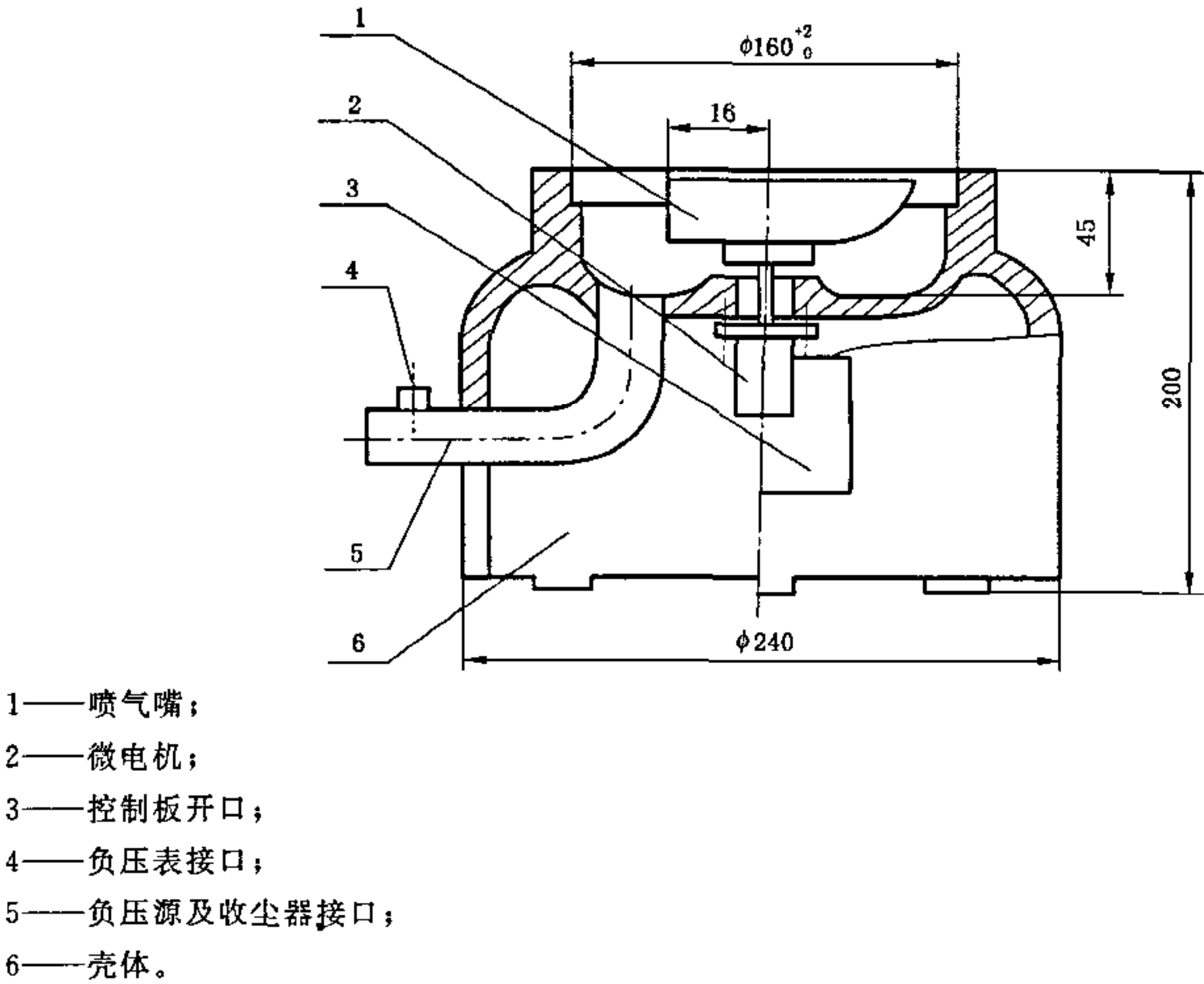
图 A.2 筛座示意图
