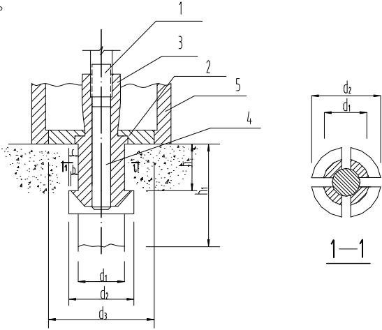
图 4.1.3-1 圆环式后装拔出法检测装置
