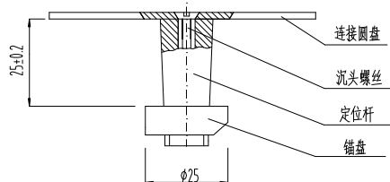
图 6.2.1 预埋件及安装
