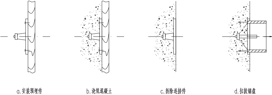
图 6.1.5 预埋拔出试验
