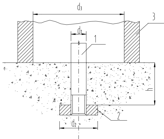
图 4.1.3-2 圆环式预埋拔出法检测装置
