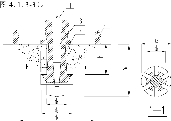
图 4.1.3-3 三点式后装拔出法检测装置
